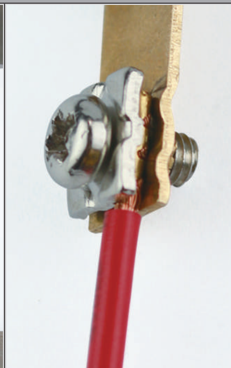
Dettaglio terminale
