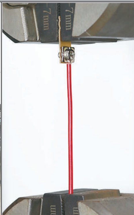
Dettaglio ganasce
